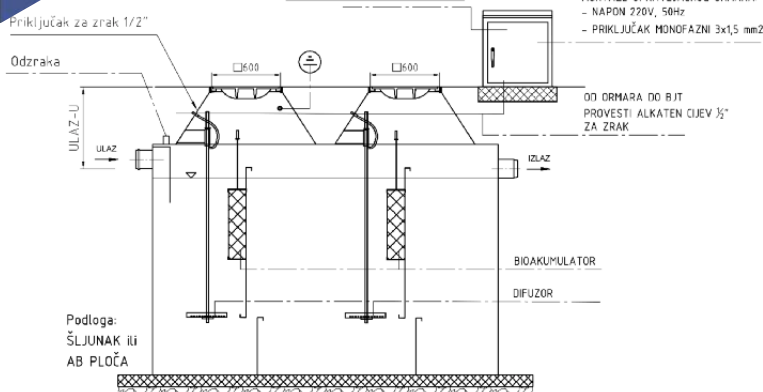
UGRADNJA BIOJAME / INSTALACION
