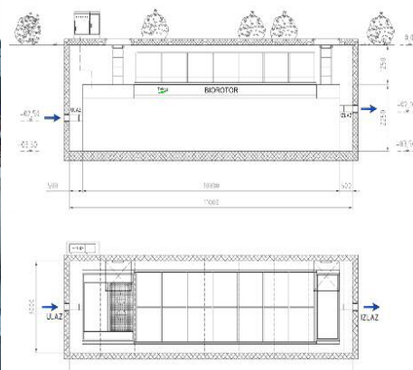
Ugradnja u betonski bazen
