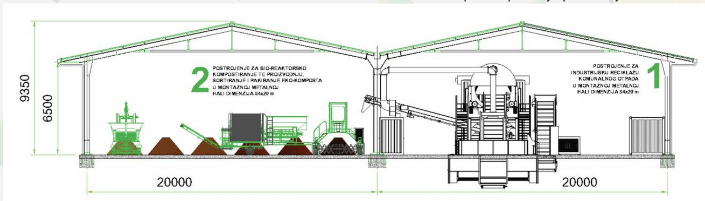
Postrojenje za bioreaktorsko kompostiranje
